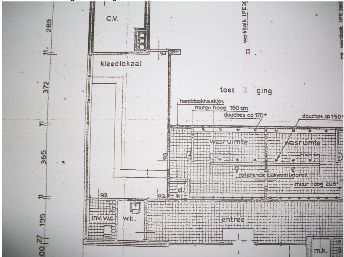
Nieuwe situatie linker gedeelte laagbouw
