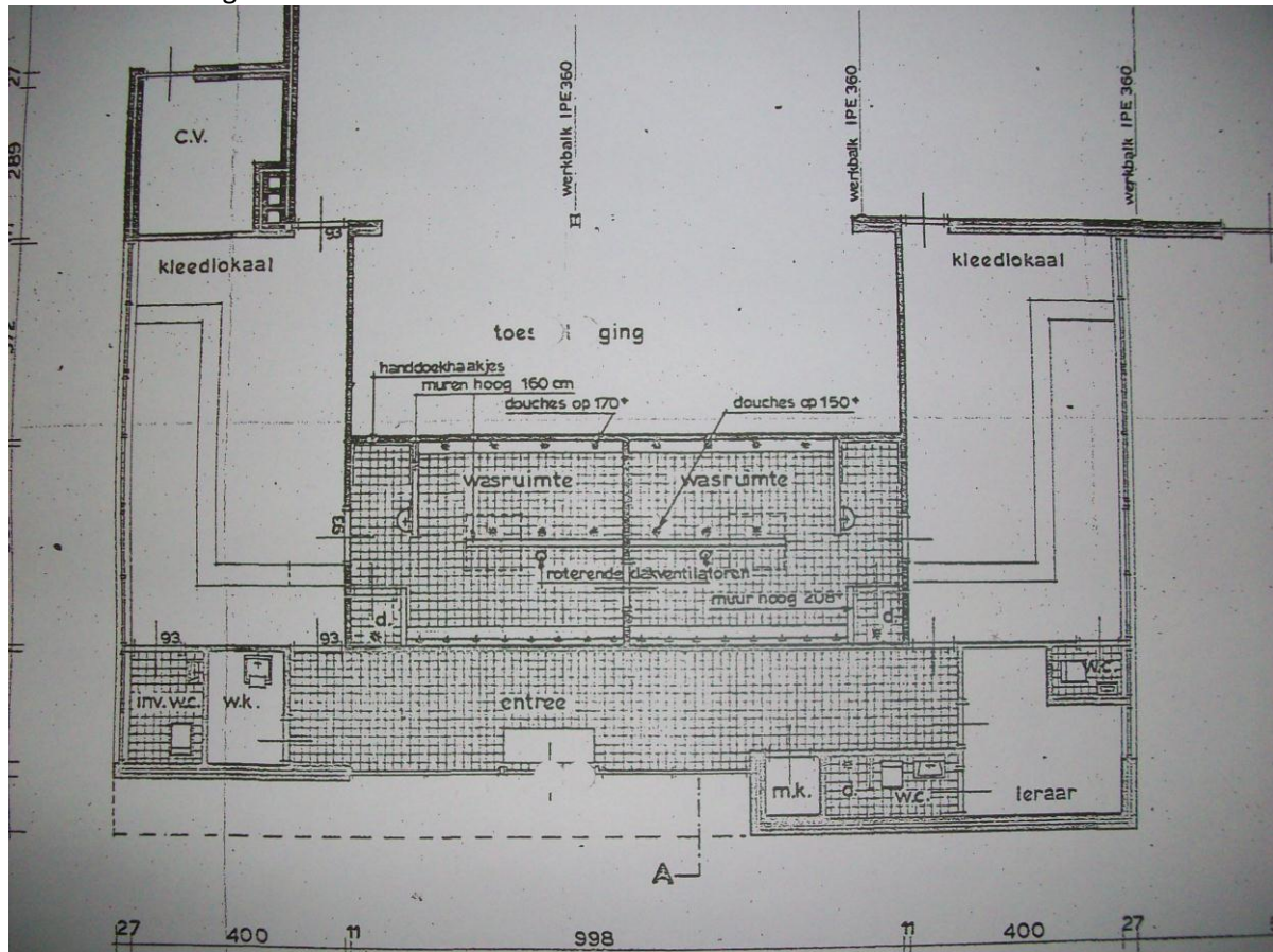
Nieuwe situatie laag bouw
